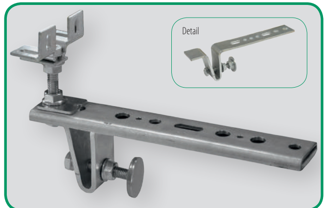
Statikgarnitur Typ Emsland mit Anschlag und Schwerlastkonsole
