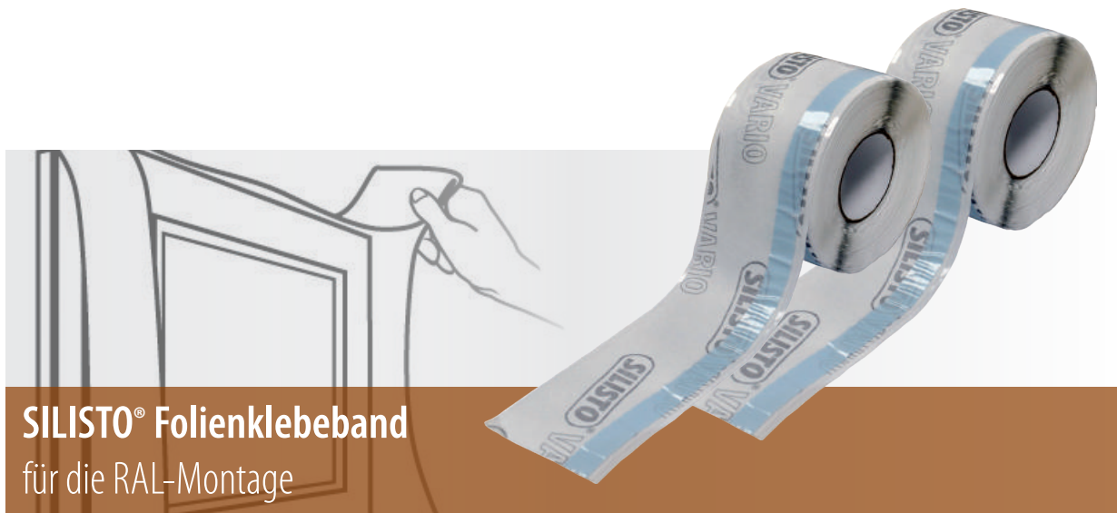
SILISTO® UFA Äußere Abdichtung für bodentiefe Fenster
