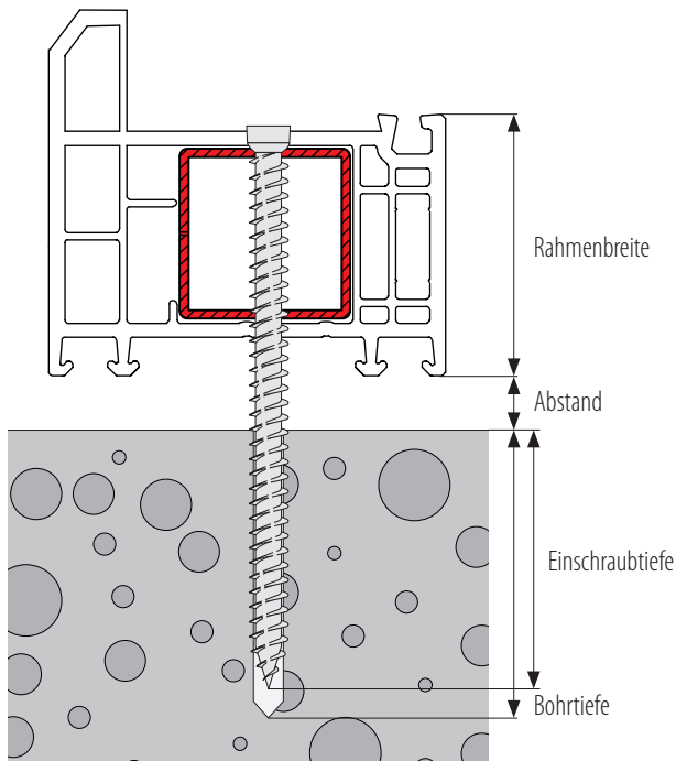
Einbaubeispiel Kunststofffenster
