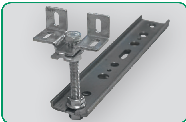
Statikgarnitur Typ Emsland mit Anschlag
